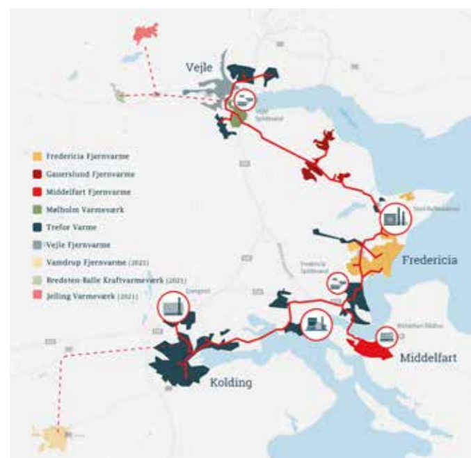
Figur 19. Varmetransmission i Trekantområdet forbinder varmeproduktion og lokale fjernvarmeområder via TVIS' fjernvarmenet (røde linjer). Kilde: TVIS.net
